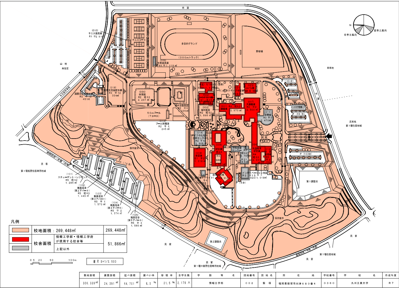
配置図
